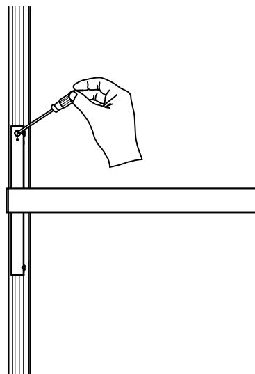
Bloquear fijación girando 90° la pieza. Block fixing by turning the piece 90°.
